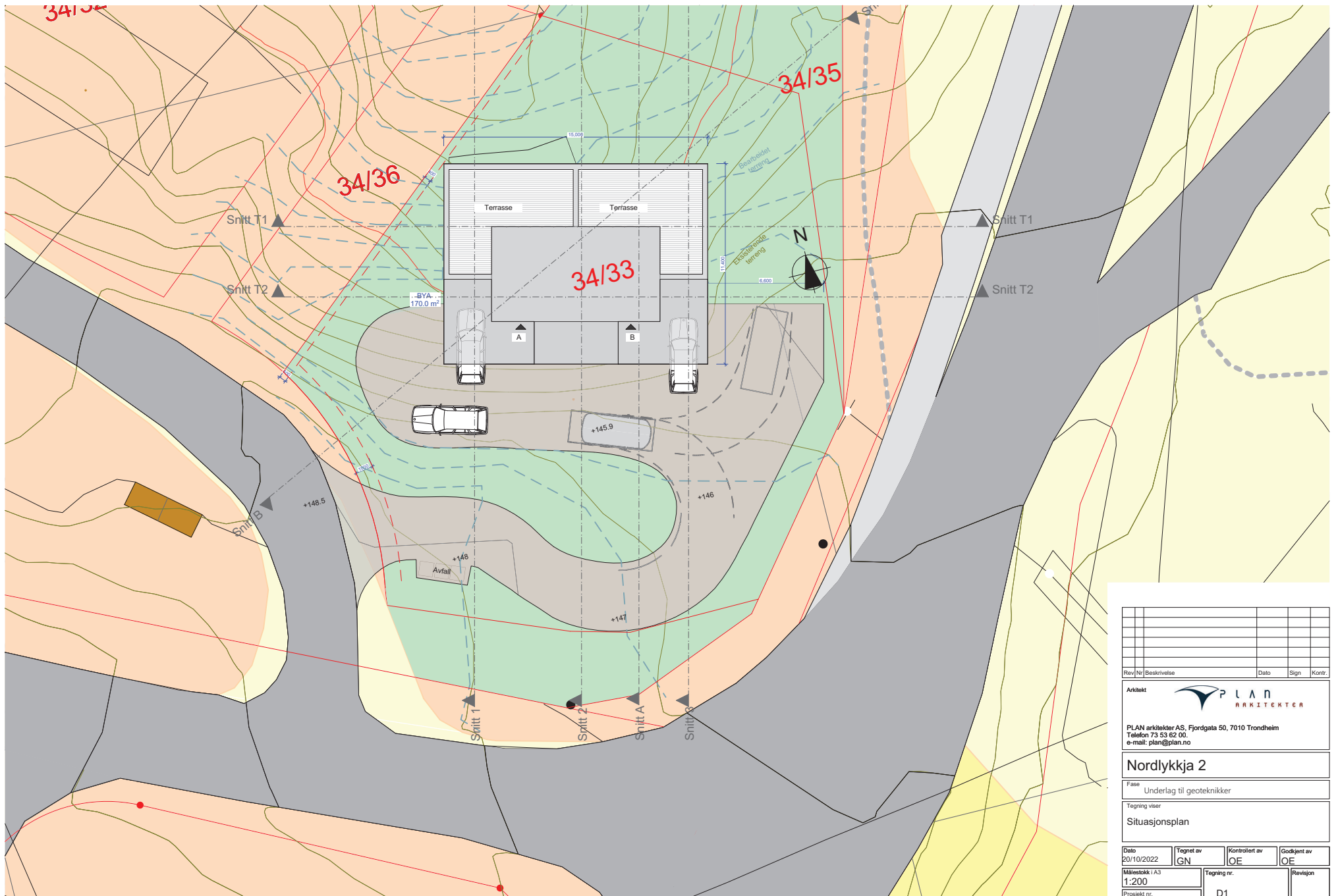
1:200 Situasjonsplan
