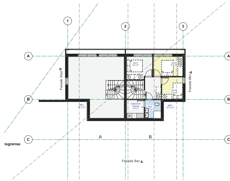
1:200 2. Etasje
