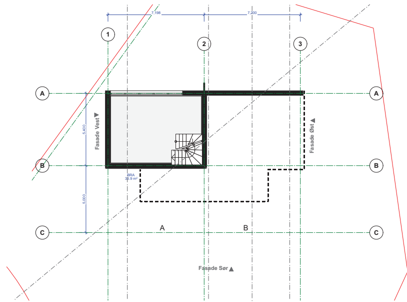
1:200 1. Etasje
