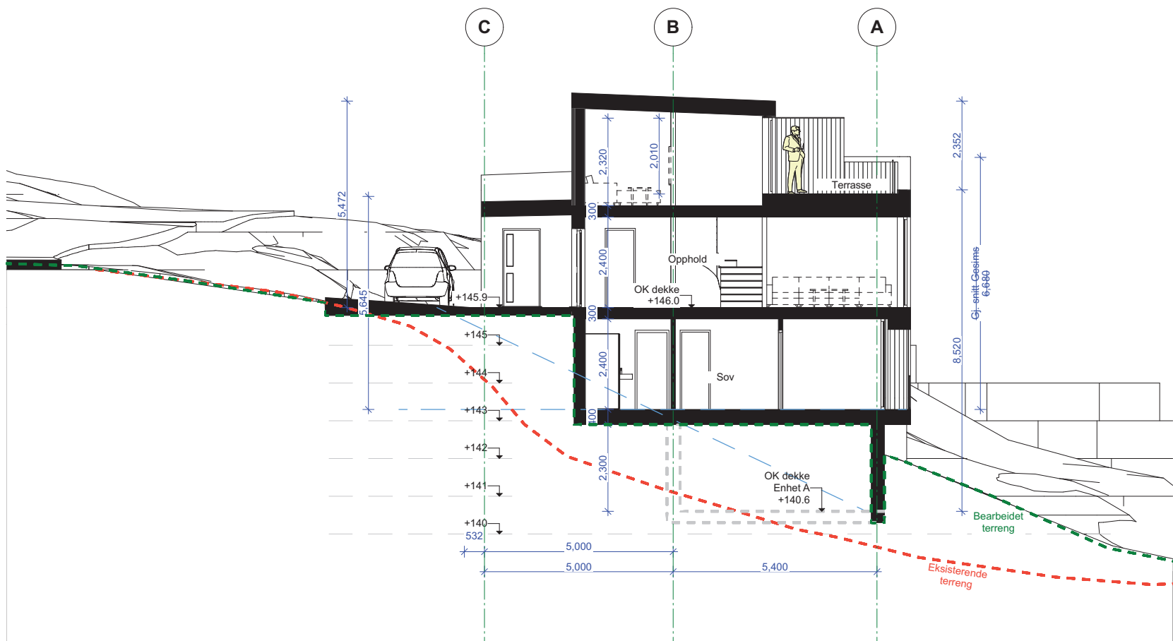
1:100 Snitt A
