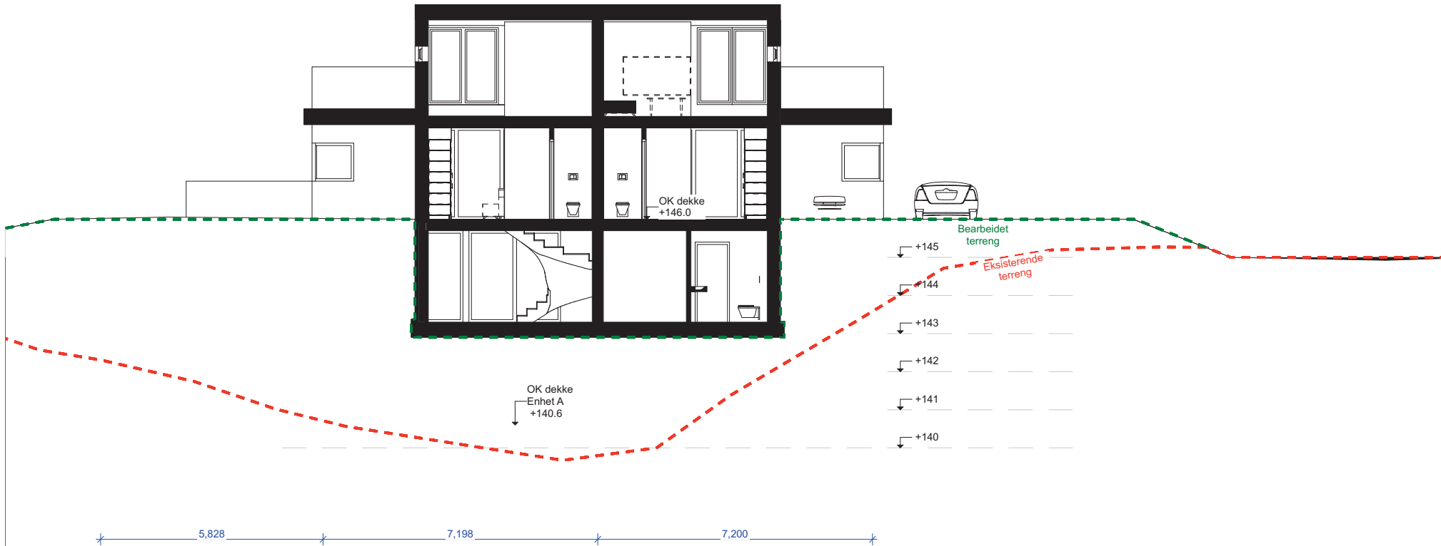
1:100 Snitt T2
